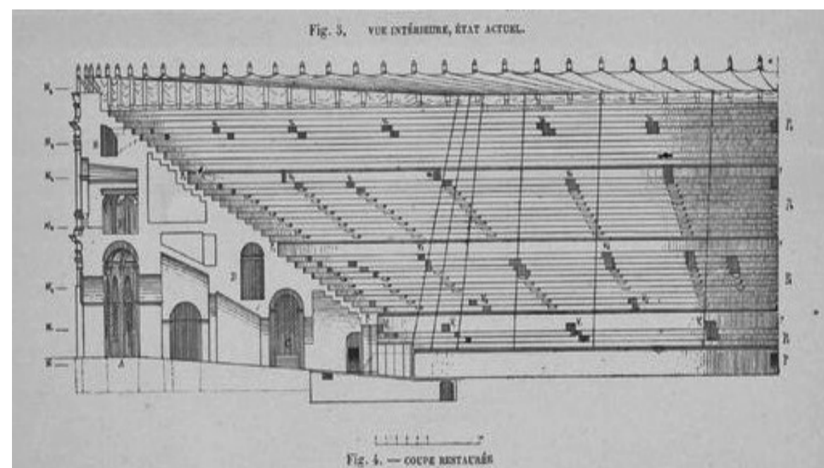
Elevación interior de la obra
