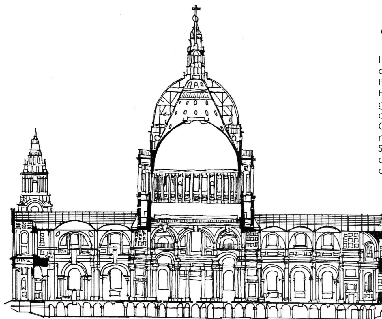
Corte longitudinal de la catedral donde aparece el gran acceso, la nave, la cúpula y el coro.
