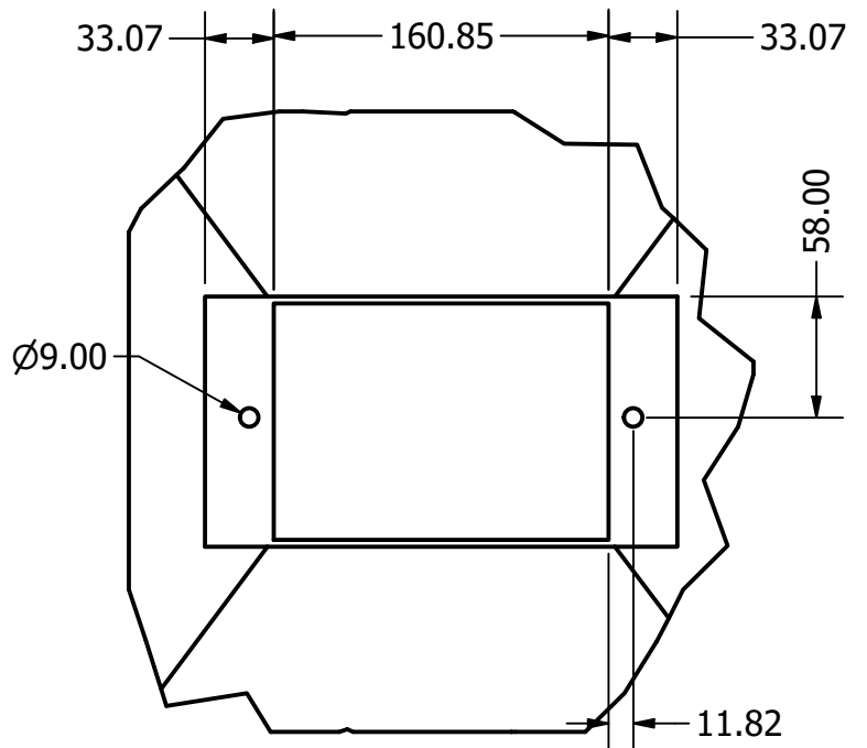
DETALLE A ESCALA 1 / 4
