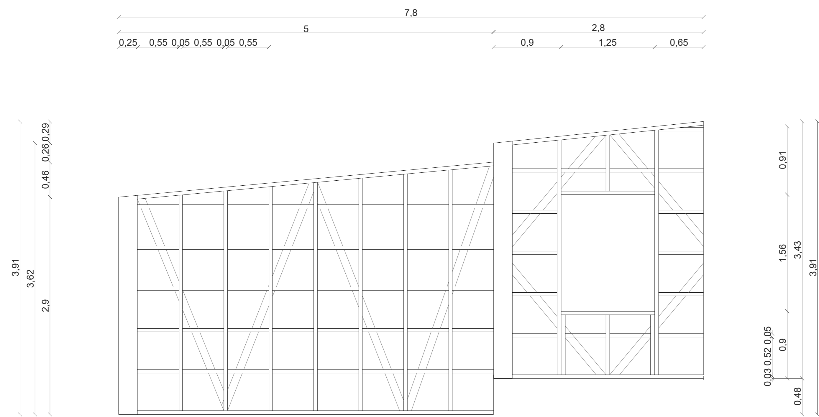
ELEVACION MURO C ESC. 1:20
