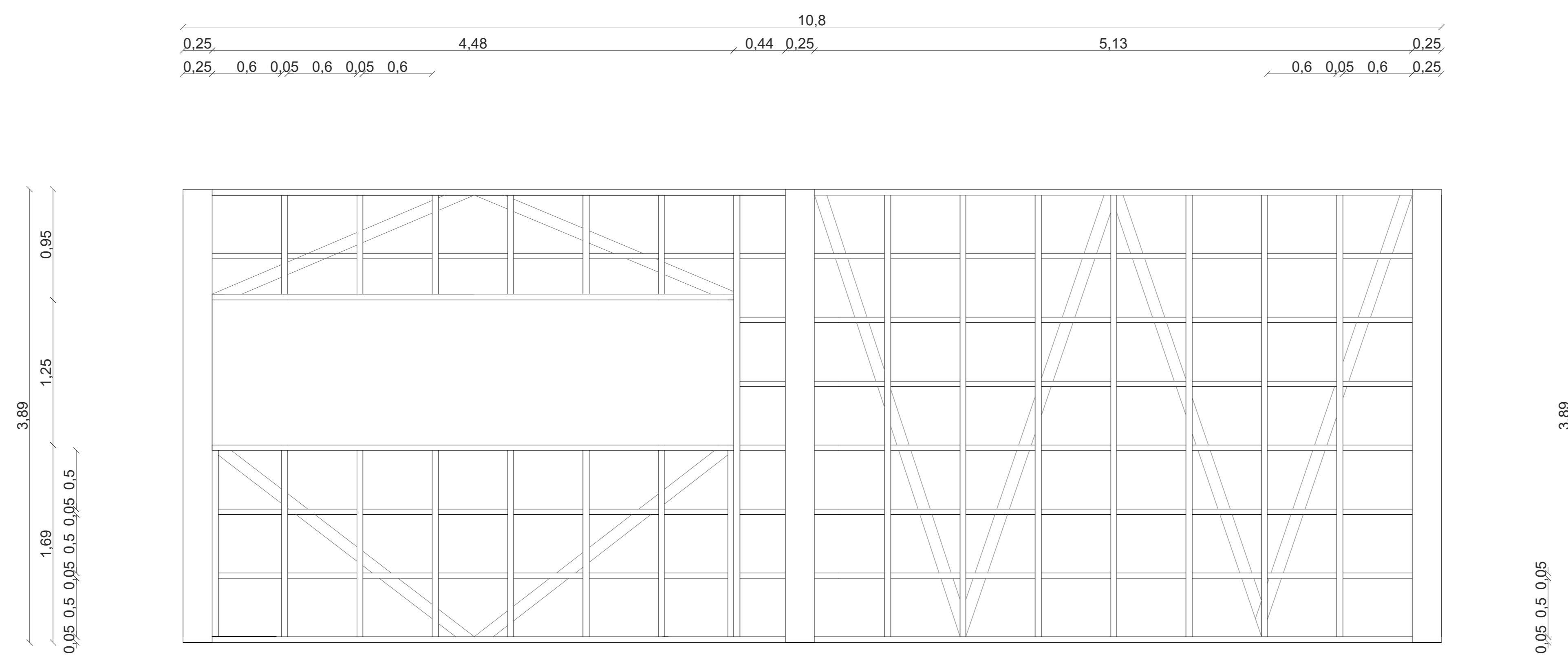
ELEVACION MURO F ESC. 1:20
