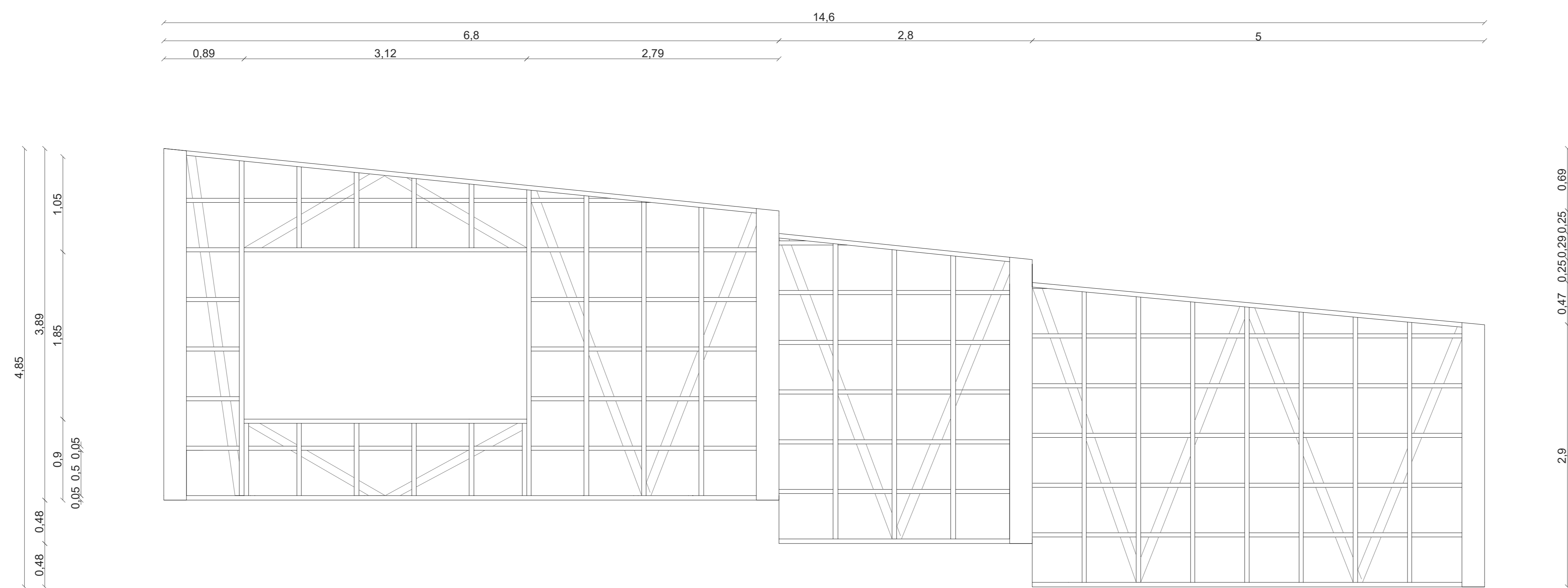
ELEVACION MURO E ESC. 1:20
