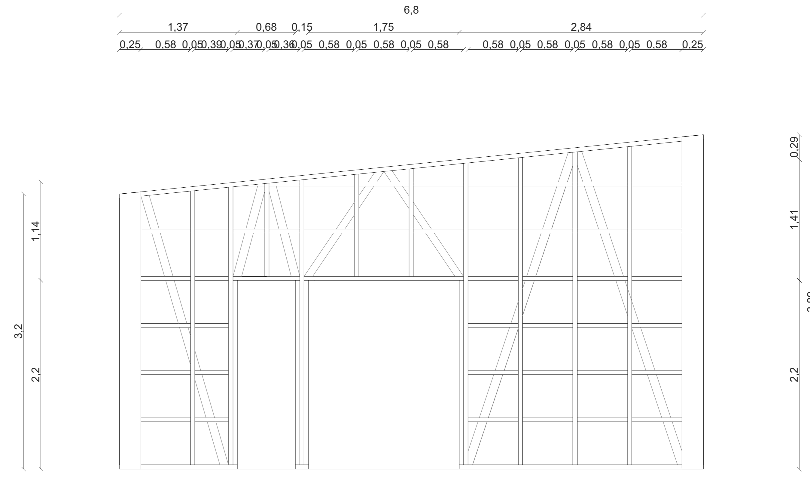
ELEVACION MURO A (NORTE) ESC. 1:20
