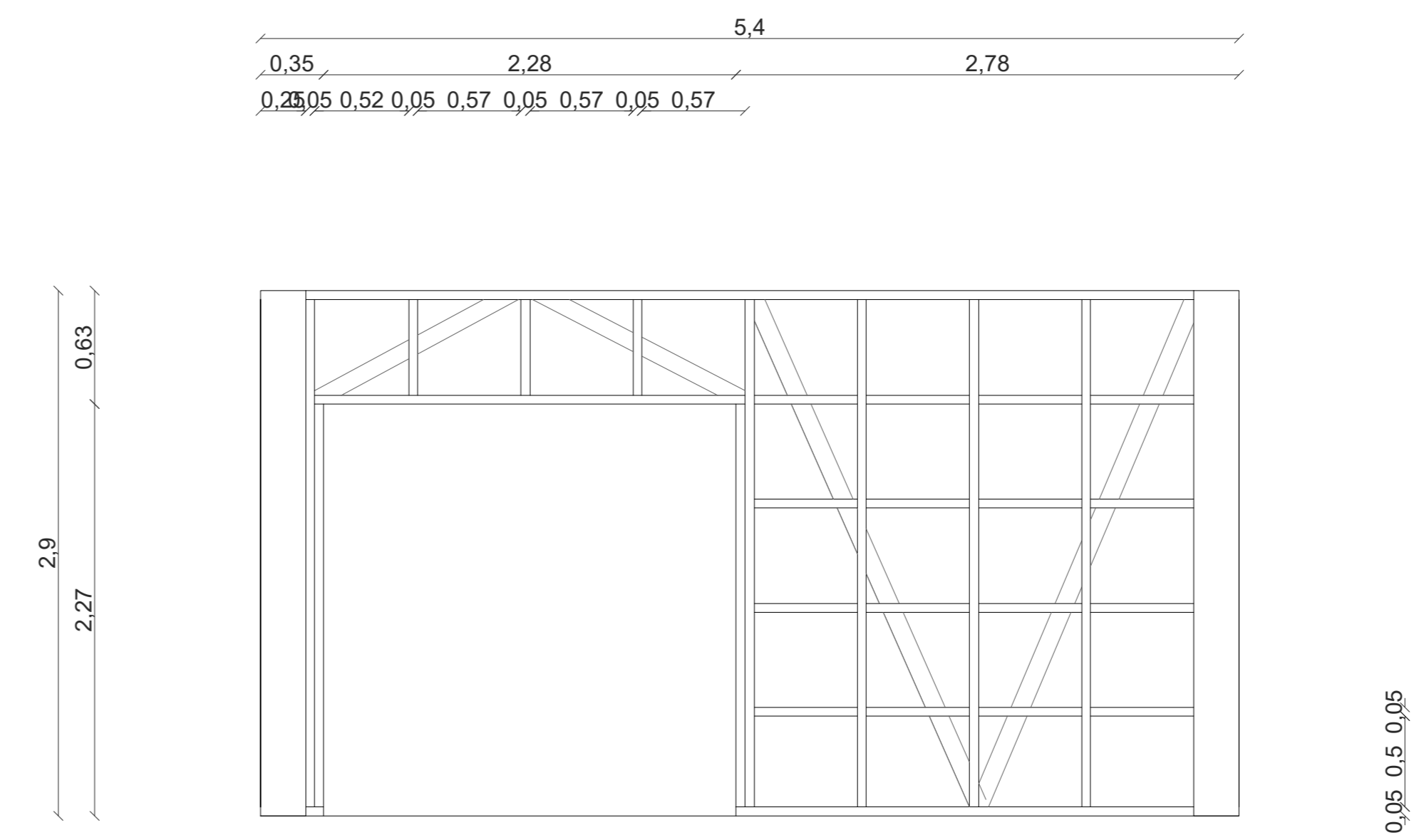
ELEVACION MURO D ESC. 1:20
