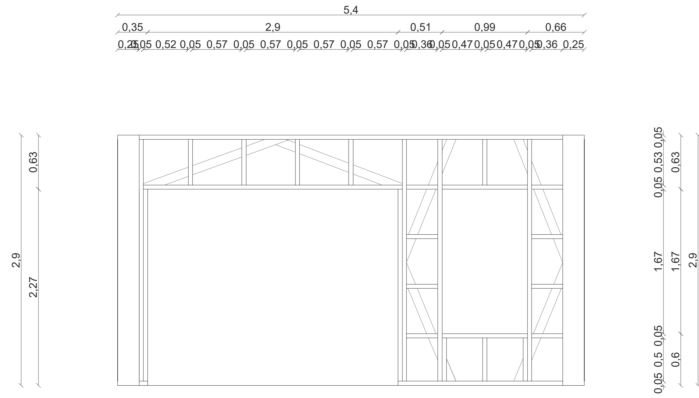
ELEVACION MURO B ESC. 1:20
