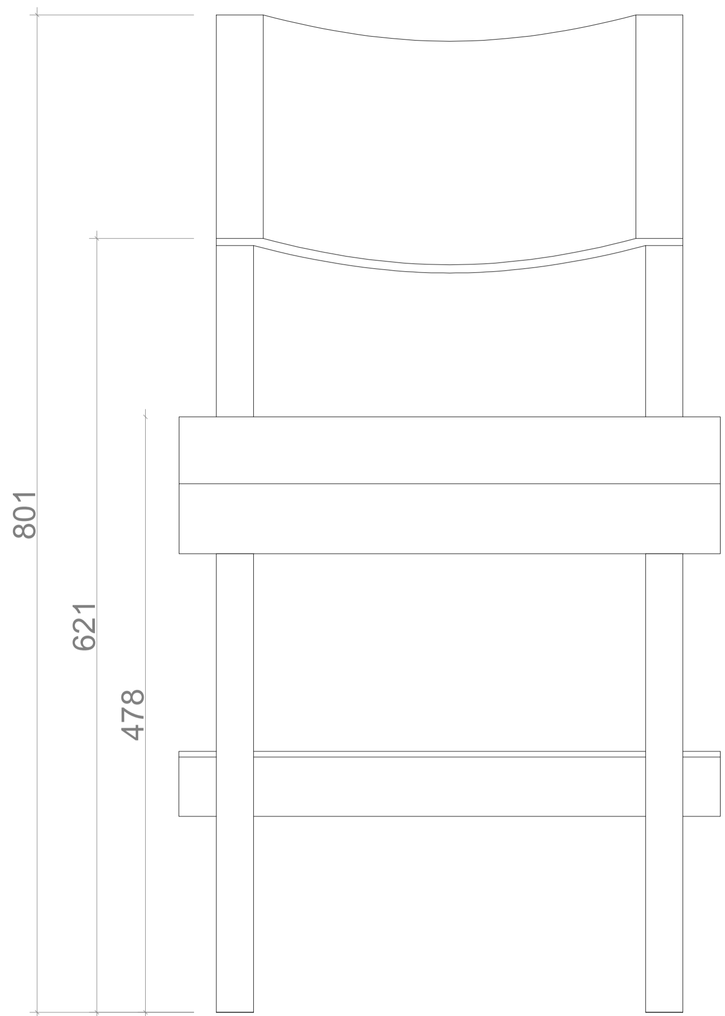
VISTA FRONTAL 1:3
