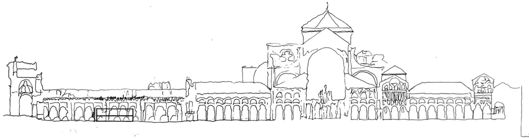
SECCION POR EL EJE DEL MIHRAB.
