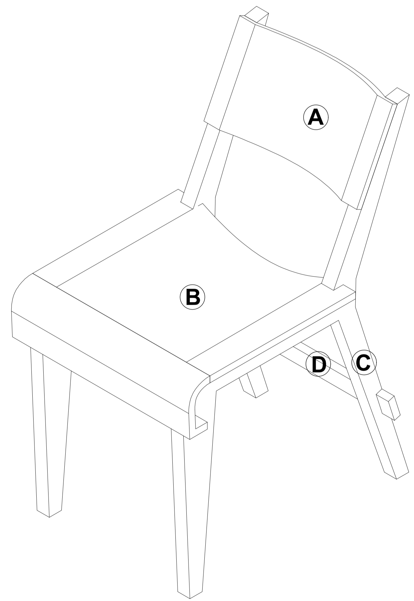
AXONOMÉTRICA GENERAL 1:4
