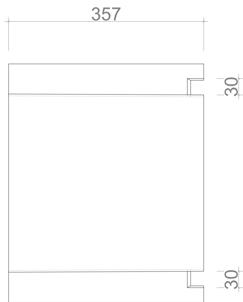
B.ASIENTO 1:4
