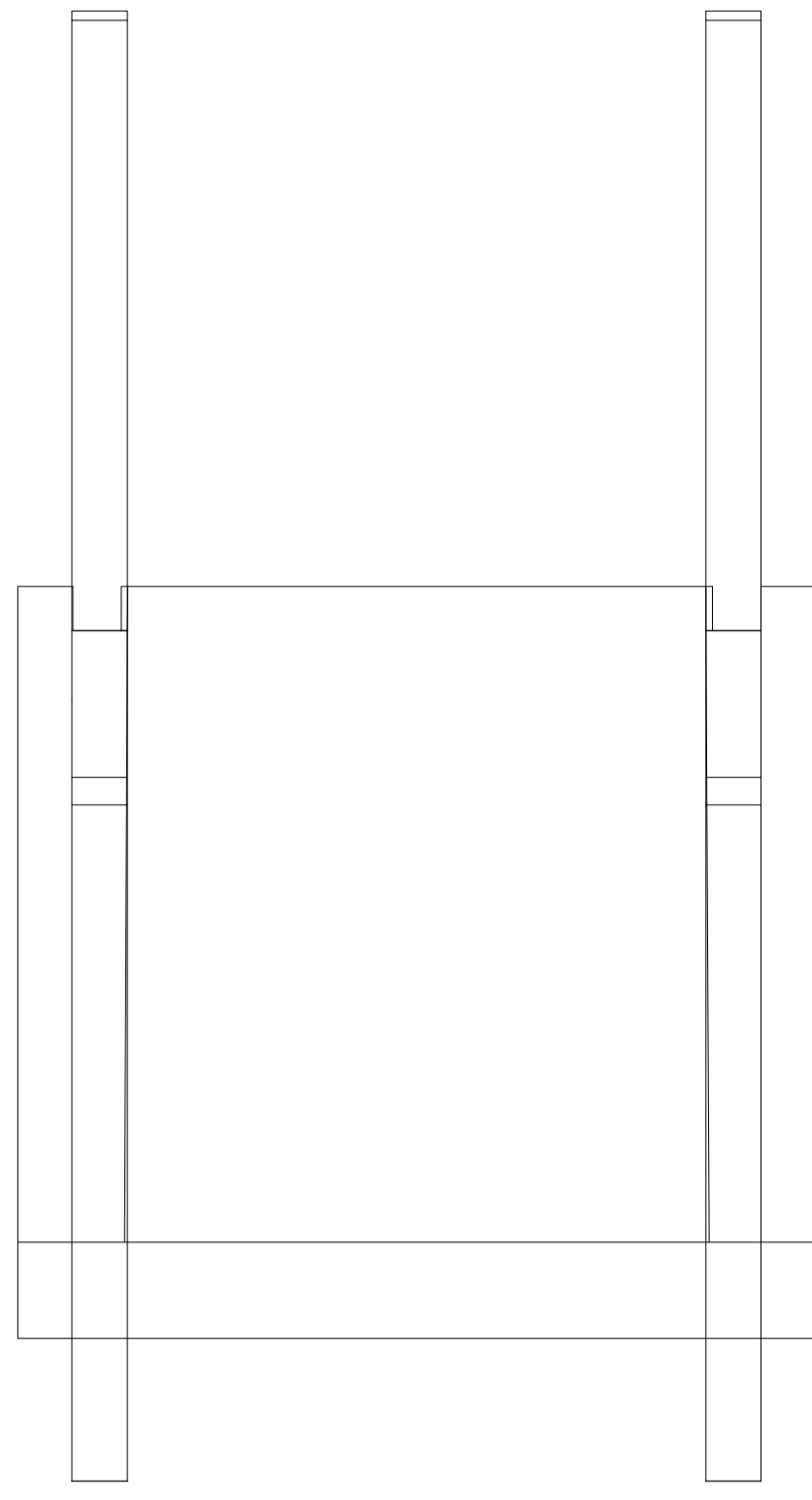
ENCAJE ASIENTO Y RESPALDO 1:4
