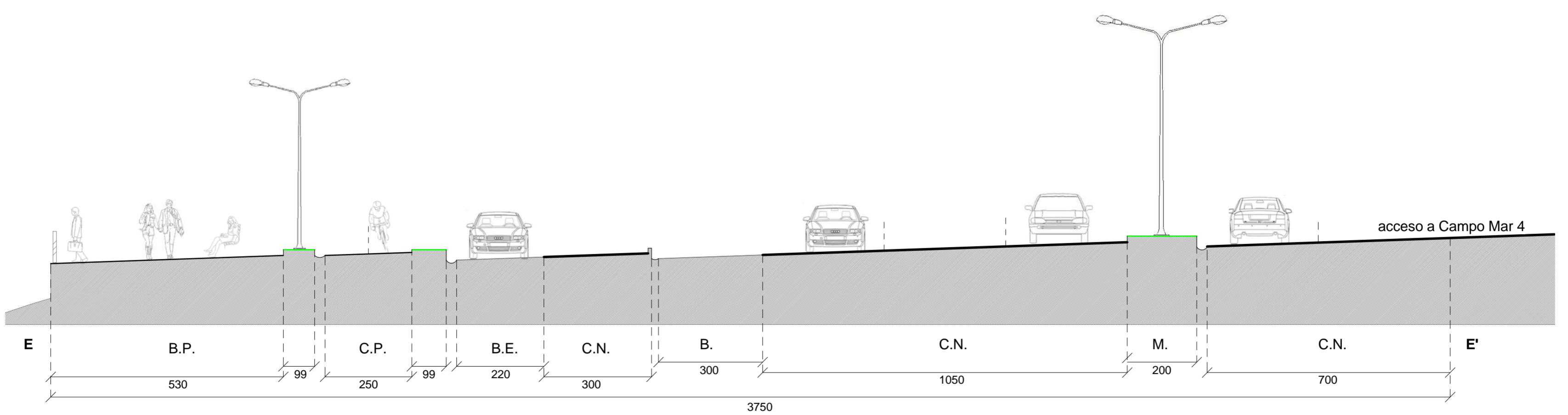
2 Corte E-E' 6 1:100
