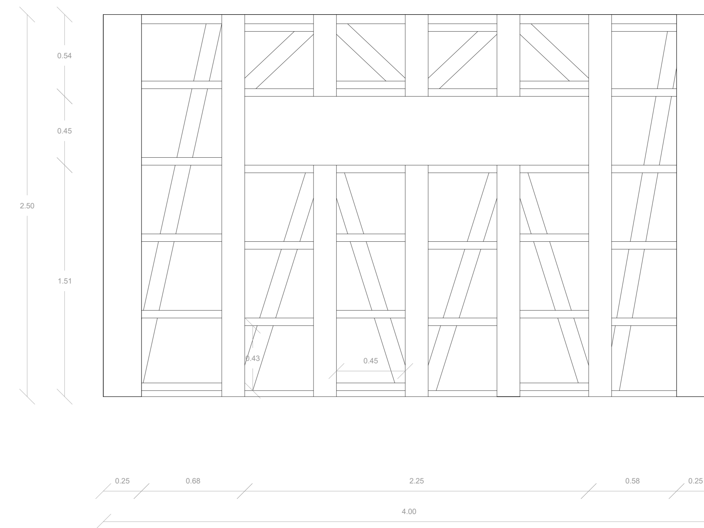
Elevación 9
