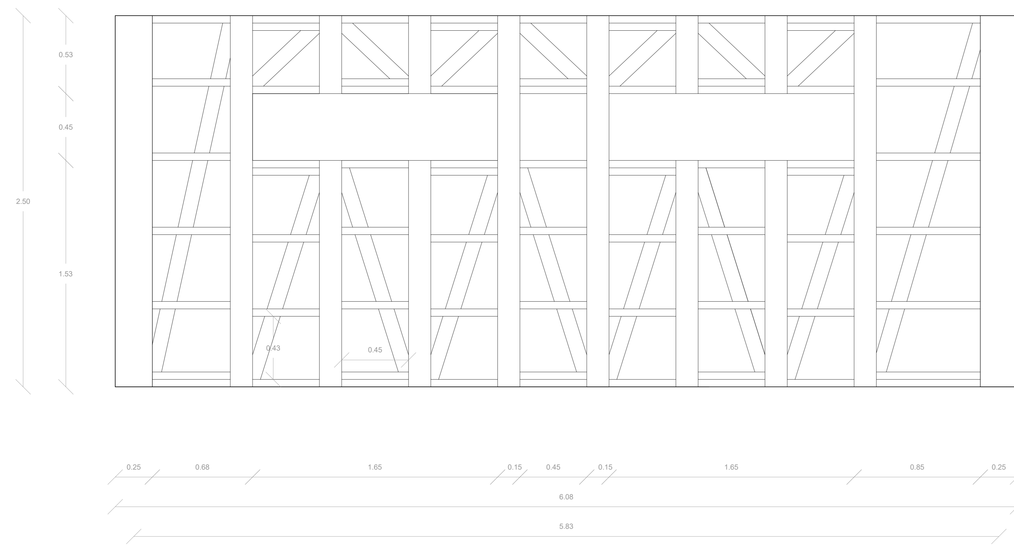
Elevación 8
