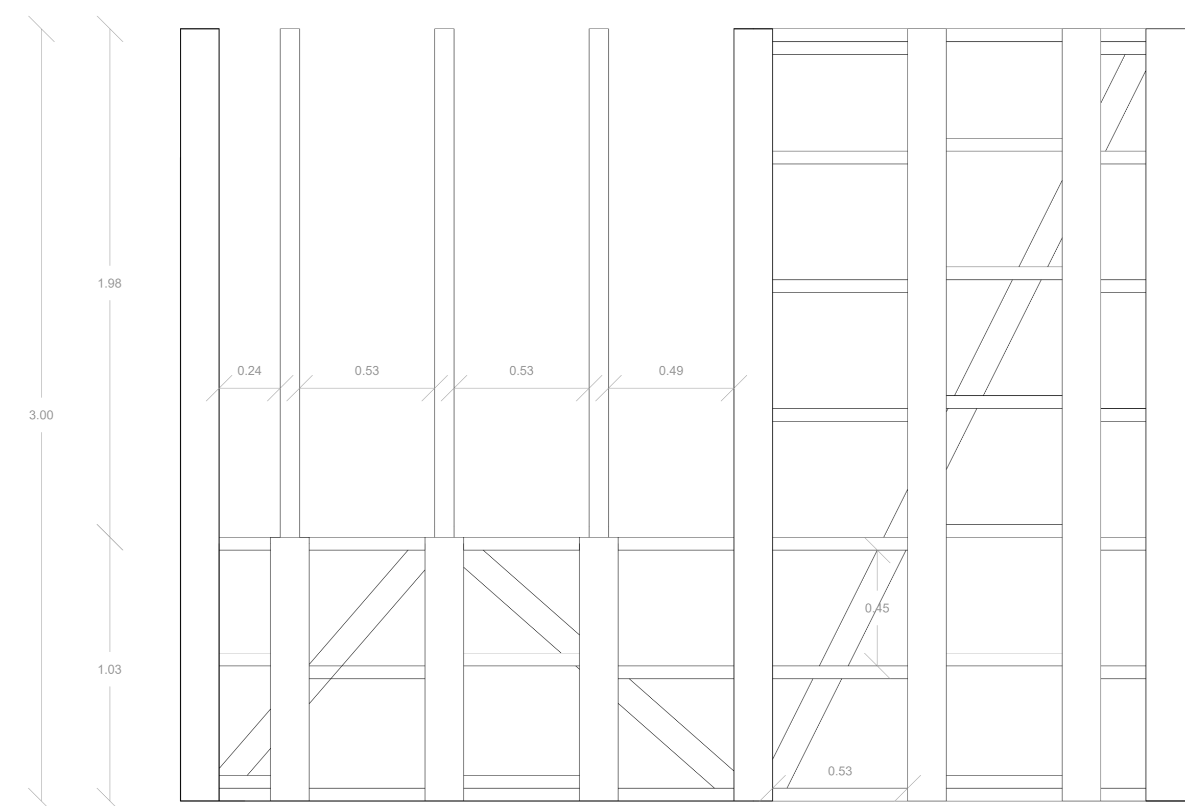
Elevación 4
