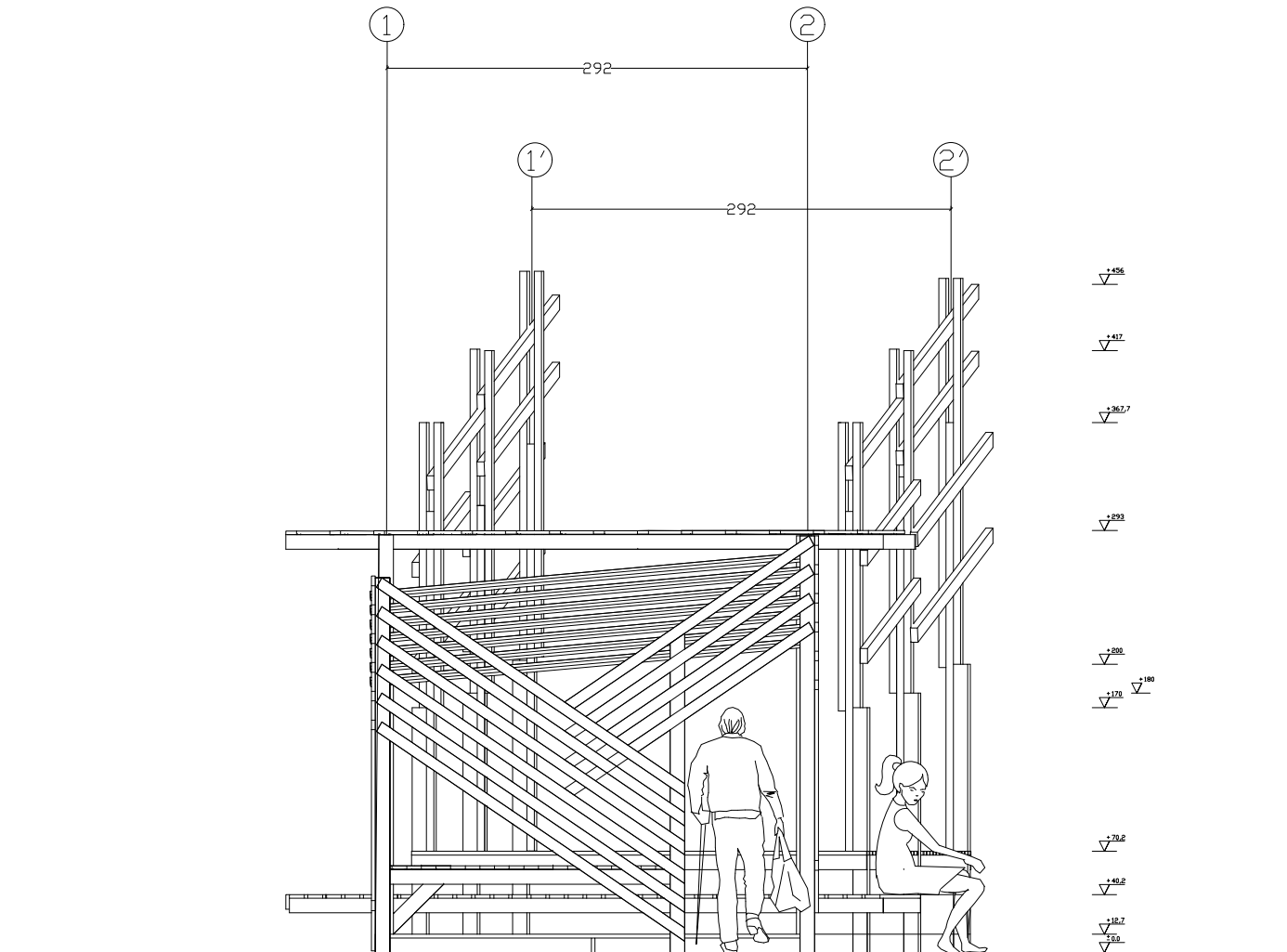
ELEVACIÓN SUR ESC. 1:200
